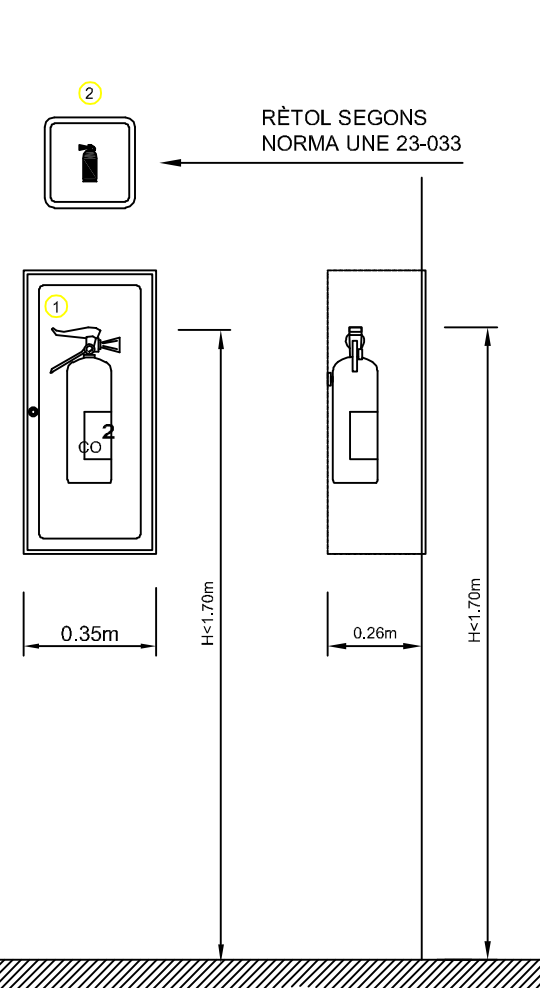
DETALL EXTINTOR CO 2 I EXTINTOR EMPOTRATS
