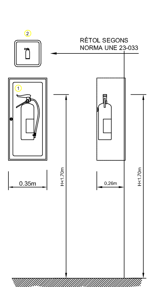
DETALL EXTINTOR EMPOTRAT
