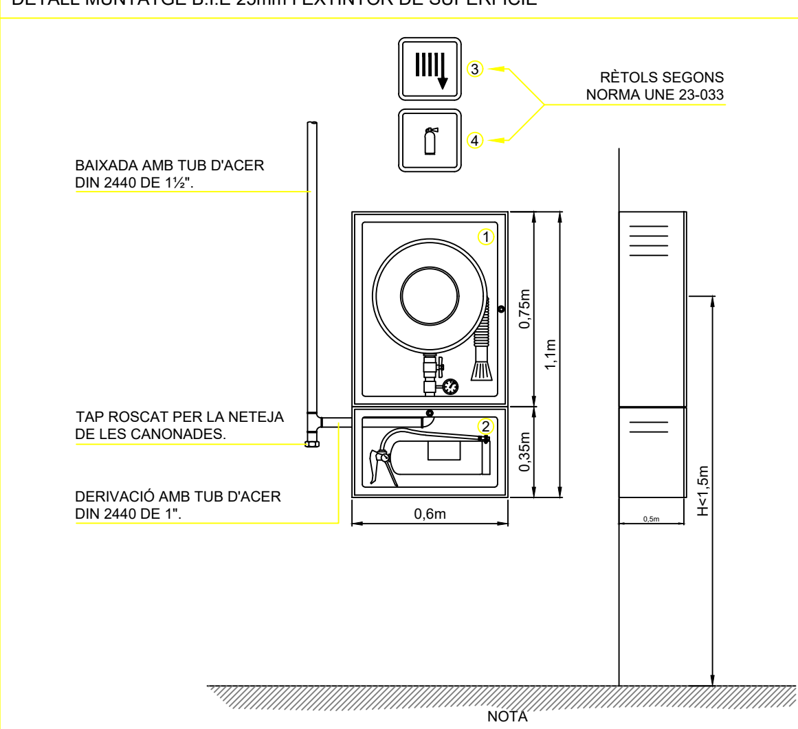
DETALL MUNTATGE B.I.E 25mm i EXTINTOR DE SUPERFÍCIE
