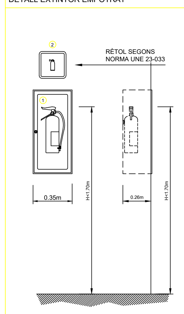
DETALL EXTINTOR EMPOTRAT
