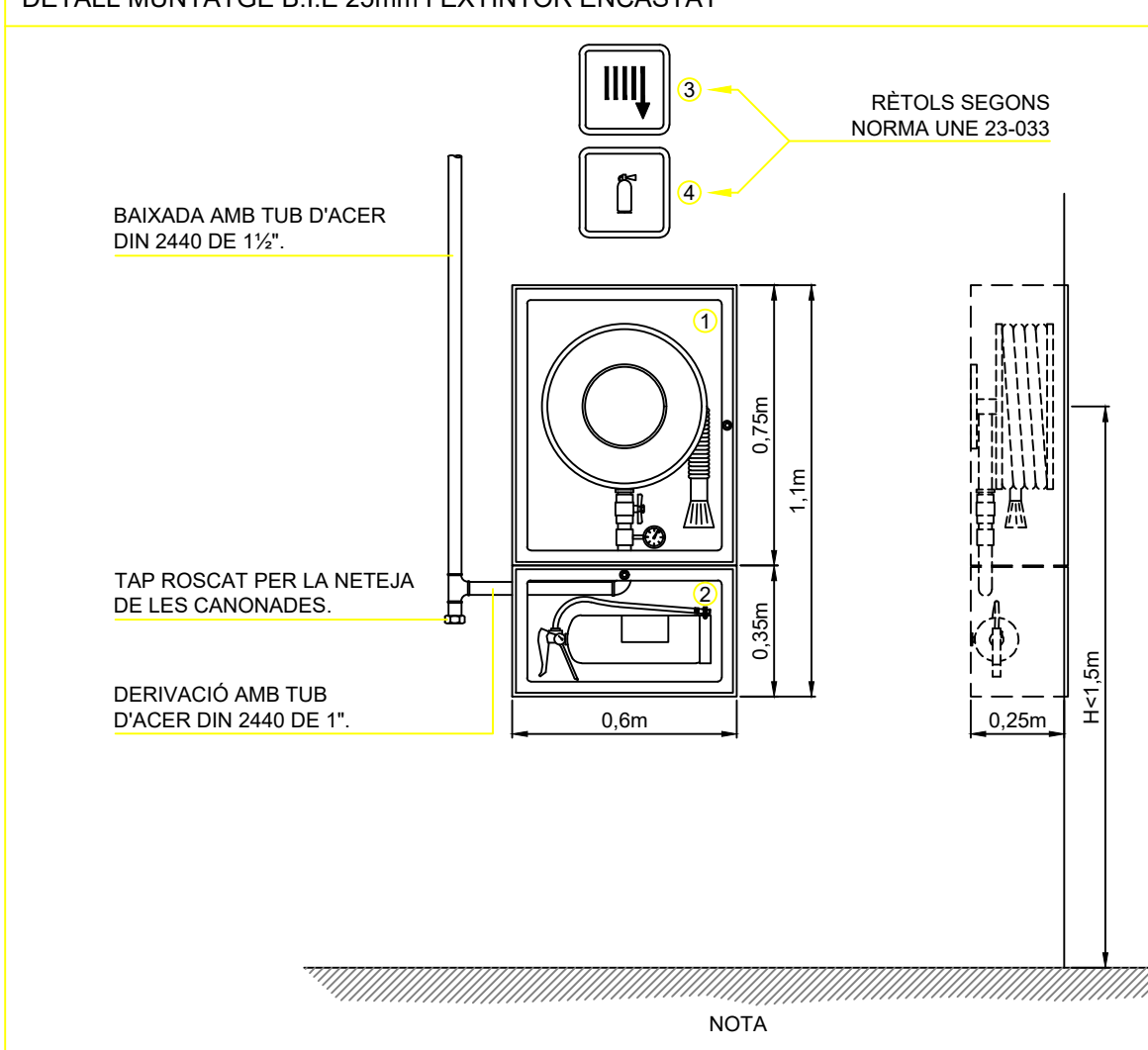
DETALL MUNTATGE B.I.E 25mm i EXTINTOR ENCASTAT
