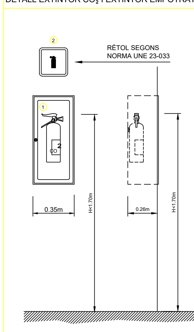
DETALL EXTINTOR CO 2 i EXTINTOR EMPOTRATS
