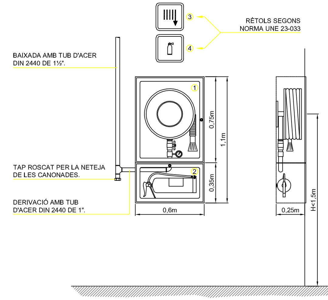
DETALL MUNTATGE B.I.E 25mm I EXTINTOR ENCASTAT
