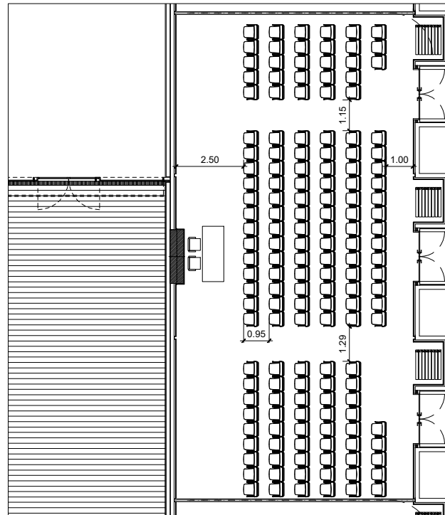
SALA REUNIONS 3+5+7 - Planta primera FORMAT TEATRE - MÀXIMA CAPACITAT Escala format A4 1:200
